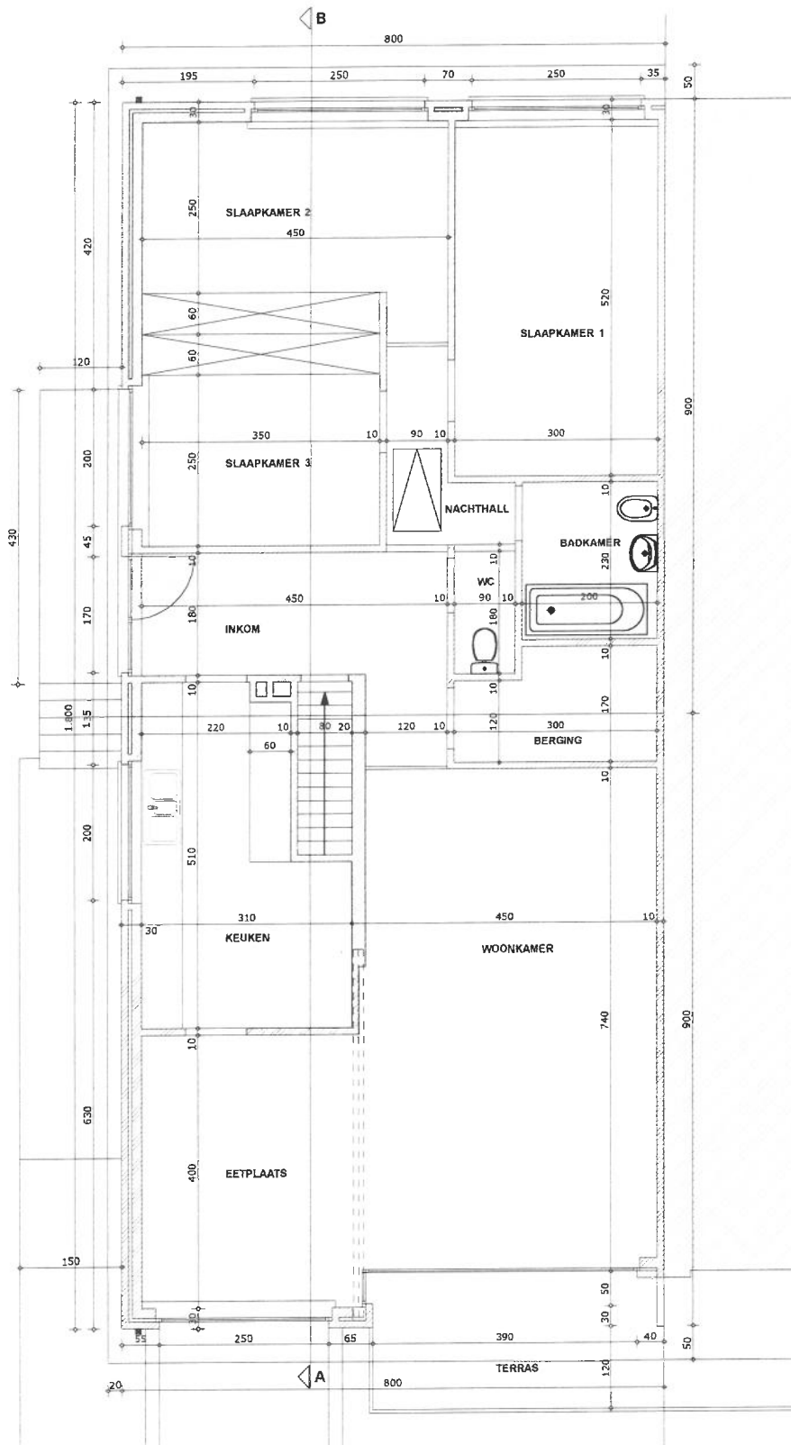
GELIJKVLOERS - BESTAANDE TOESTAND
